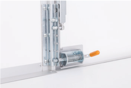
Sivuluukku lukitaan sisäpuolelta molemmista reunoista lukitustankoilla.
